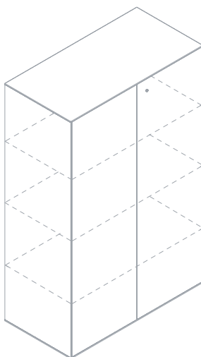
Contenitore con ante e serratura (3 ripiani) 1BA6085: L 80 P 45 H 157,7
